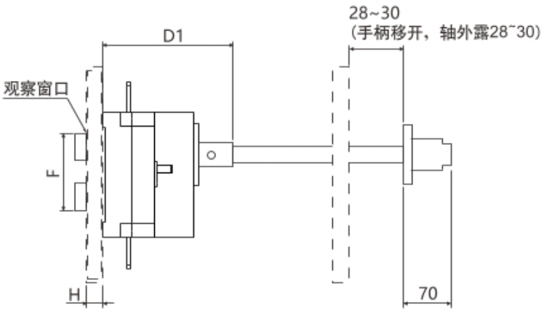
SKG1-125~630A柜外操作
