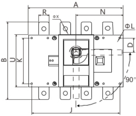
SKG1-125A~630A直接操作
