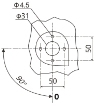
柜外手柄座安装尺寸
