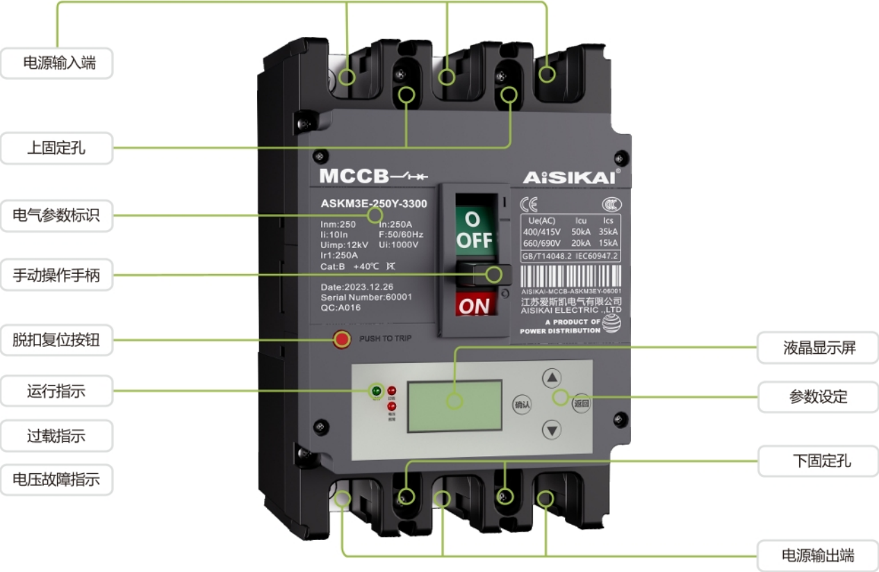
● 开关外部图
