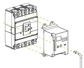
电动操作机构操作
